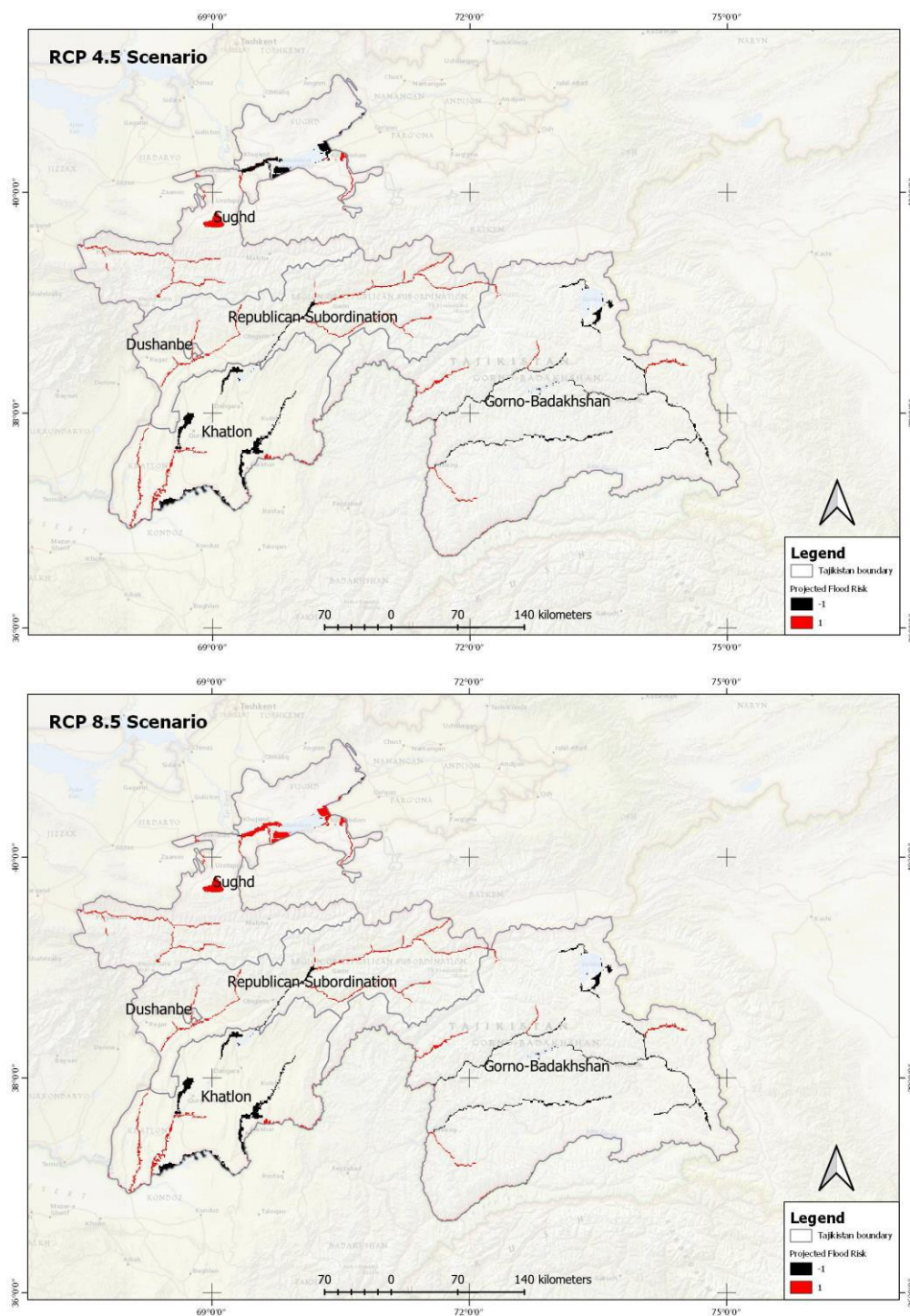
Рисунок 56: Прогнозируемое изменение риска паводков к 2050 г. с периодом повторяемости 50 лет. Прогнозы основаны на Глобальной циркуляционной модели CMIP5 для сценариев RCP 4.5 и 8.5. Карта паводков получена с учетом разницы между картой паводков RCP и картой исторических паводков.
