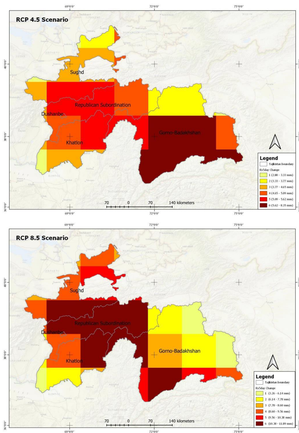
Рисунок 55: Зона риска паводков основана на изменении в 5-дневных осадках к 2050 г. Прогнозы основаны на Глобальной циркуляционной модели CMIP5 для сценариев RCP 4.5 и 8.5. Rx5day соответствует годовому максимуму 5-дневных осадков.
