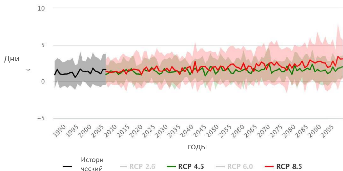
Рисунок 19: Зарегистрированное количество дней с сильными дождями Vey (20 мм / день) каждый год в 1986-2005 гг. И прогнозируемые значения на 2020-2100 гг. По всем RCP ансамблевым моделированиям CIMP5.
