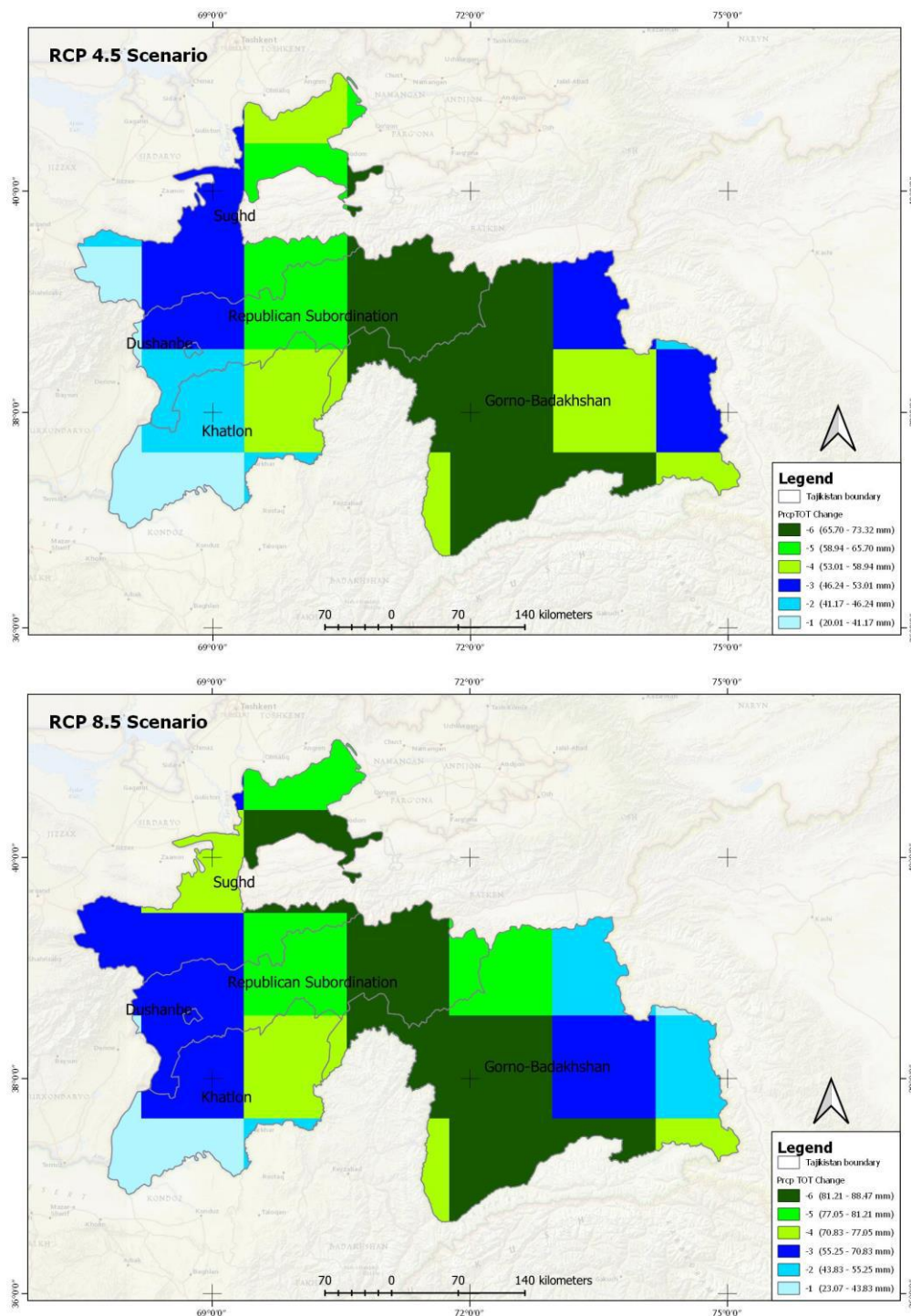
Рисунок 34: Прогнозируемое изменение общего количества осадков к 2050 г. по сравнению с базовым за 1960-1990 гг. Прогнозы основаны на Глобальной циркуляционной модели CMIP5 для сценариев RCP 4.5 и 8.5.
