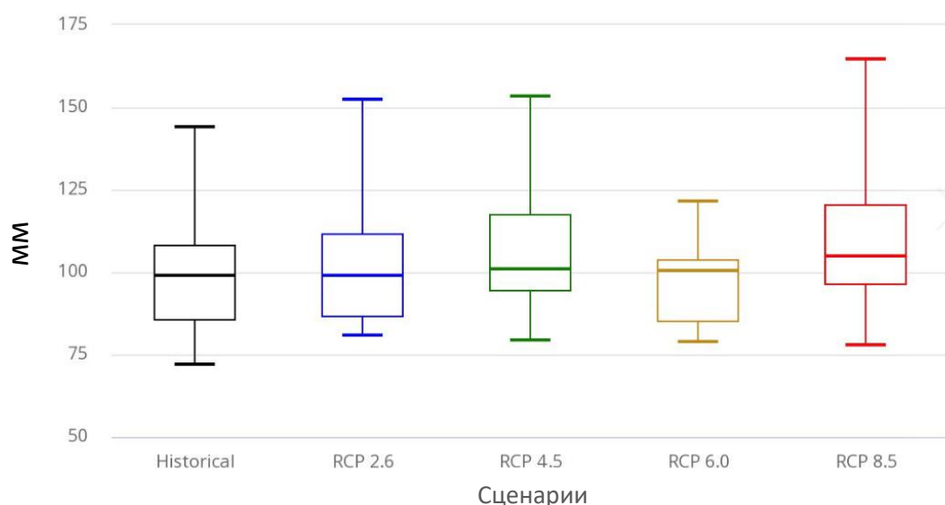
Рисунок 20: График показывает зарегистрированное 5-дневное кумулятивное количество осадков за 1986–2005 гг. и прогнозируемый 5-дневный кумулятивный уровень осадков за 25 лет к 2050 году согласно всем сценариям RCP ансамбля моделей CIMP5. Этот индикатор показывает максимальное кумулятивное за 5 дней количество осадков, которое может ожидаться за 25-летний период
