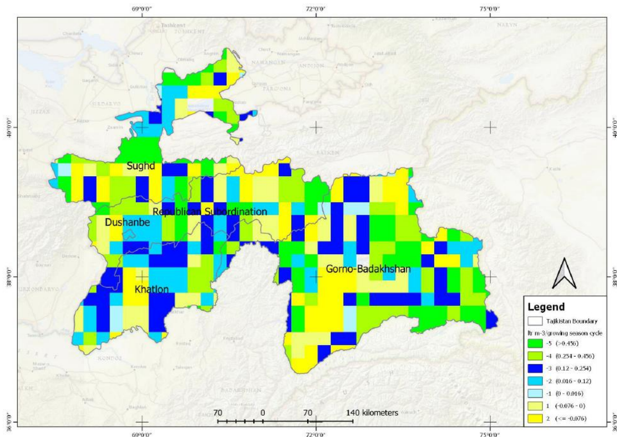
Рисунок 51: Изменение объемной поверхностной влажности почвы за 1999-2019 гг. Данные EU Copernicus и USGS. Набор данных по влажности почвы создан в рамках проекта Инициативы по изменению климата (CCI) Европейского космического агентства (ESA) по основным климатическим переменным.
