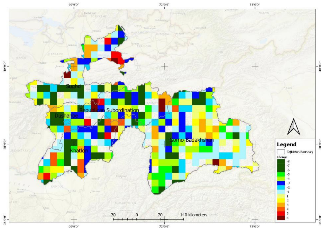
Рисунок 52: Тенденция NDVI – Динамика влажности почв в период вегетации. Данные MODIS / NASA и EU Copernicus / ESA. Классифицированная карта тенденций влажности почв в течение вегетационного периода была получена из классифицированной карты трендов NDVI
